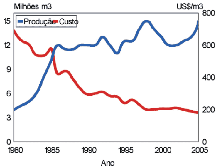
Figura 1.2: Produção e custo do etanol no Brasil.
